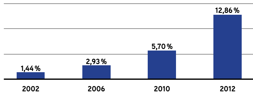
Diagram 1. Sverigedemokraternas väljarstöd 2002–2014.
